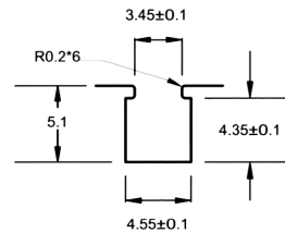
沟槽尺寸图
